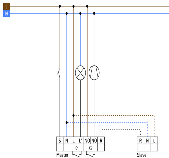
Схема подключения
