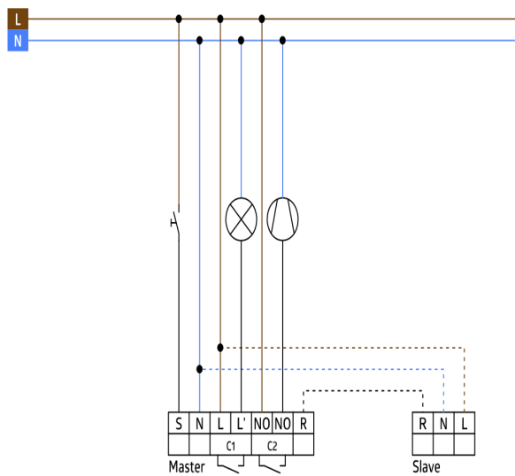
Схема подключения
