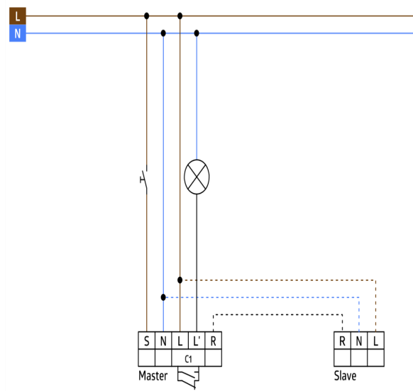
Схема подключения
