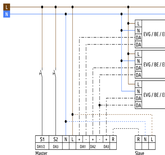
Схема подключения
