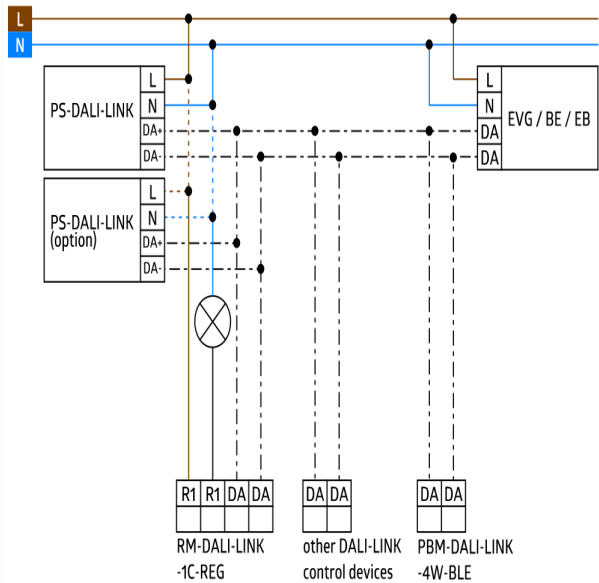
Схема подключения
