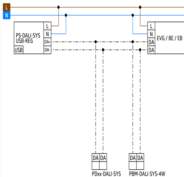
Схема подключения
