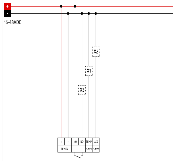
Схема подключения
