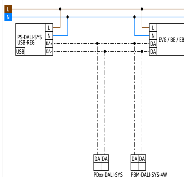
Схема подключения
