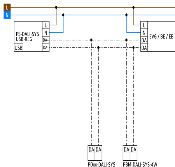
Схема подключения
