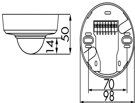
Размеры 92154
