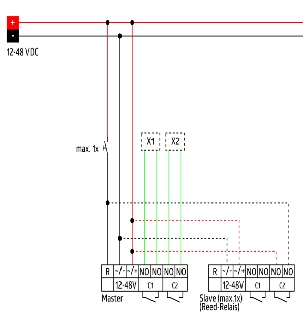
Схема подключения
