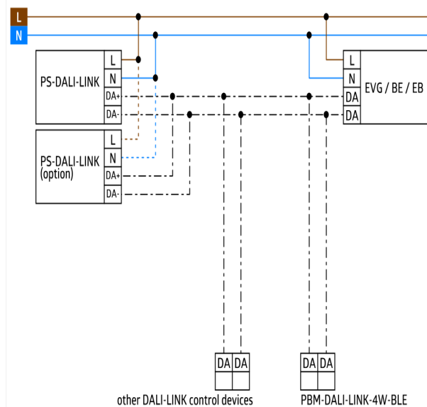
Схема подключения
