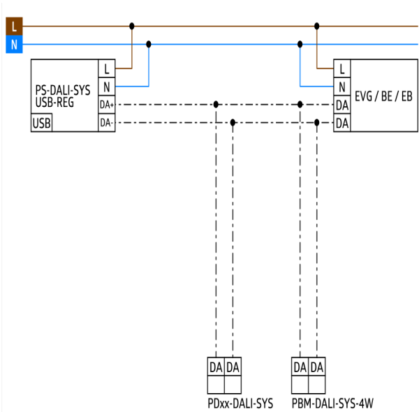
Схема подключения
