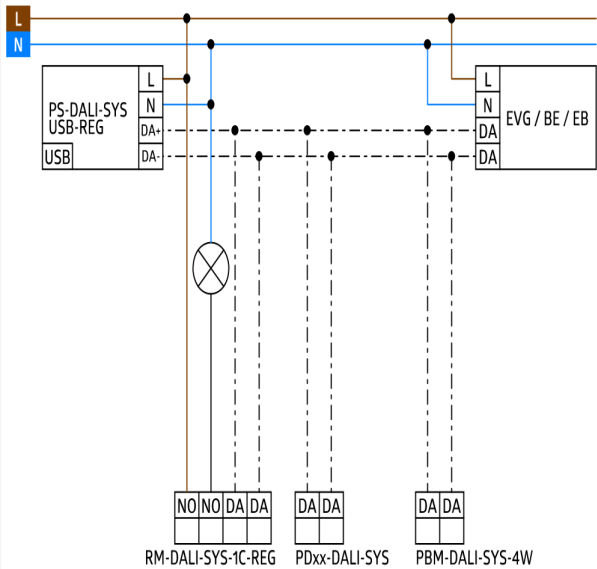
Схема подключения
