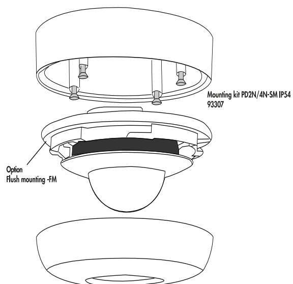
Версия для накладного монтажа (SM)
