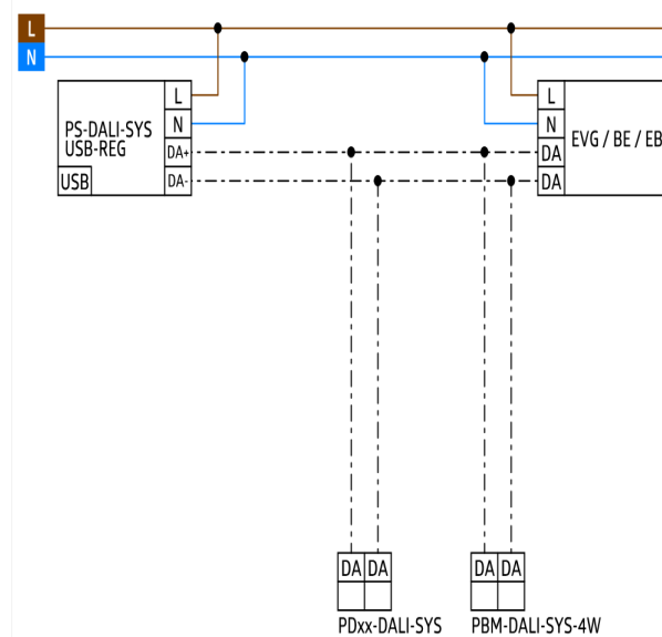
Версия для накладного монтажа (SM)
